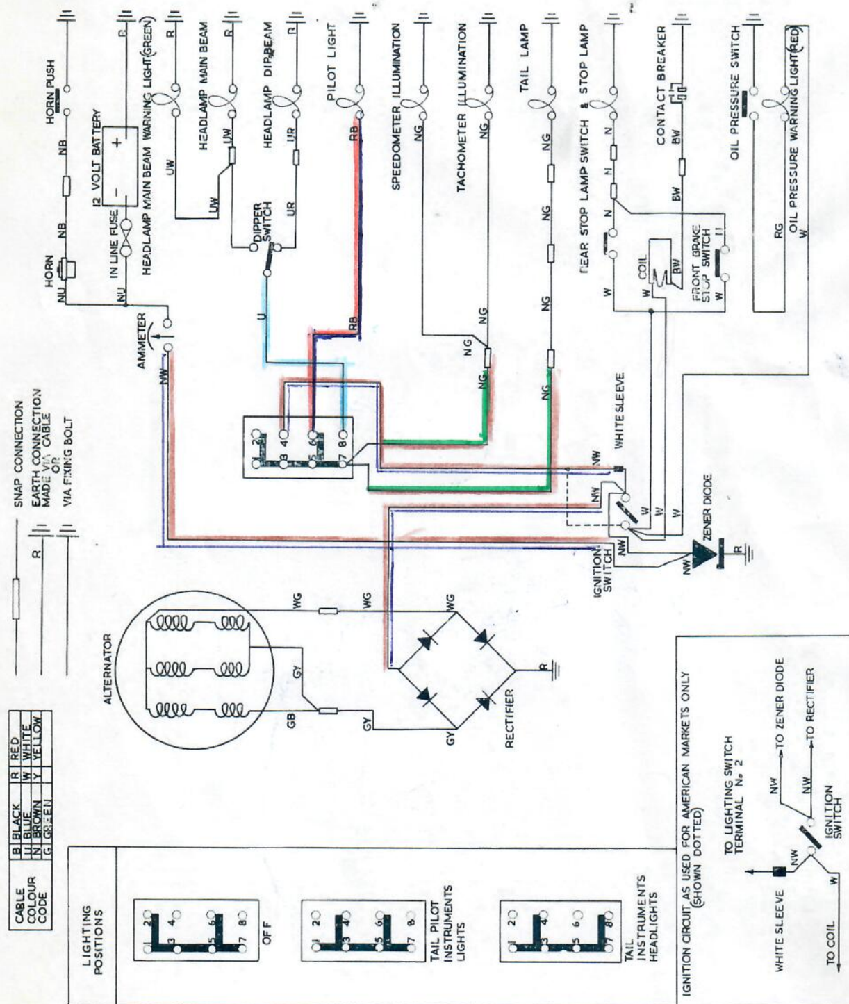
FIG. G13. Wiring diagram.
